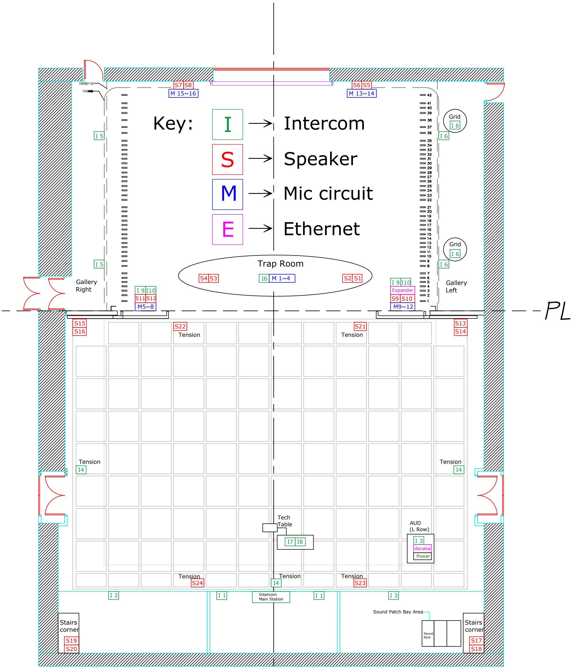
展演中心 戲劇廳 音響迴路圖 20200908
